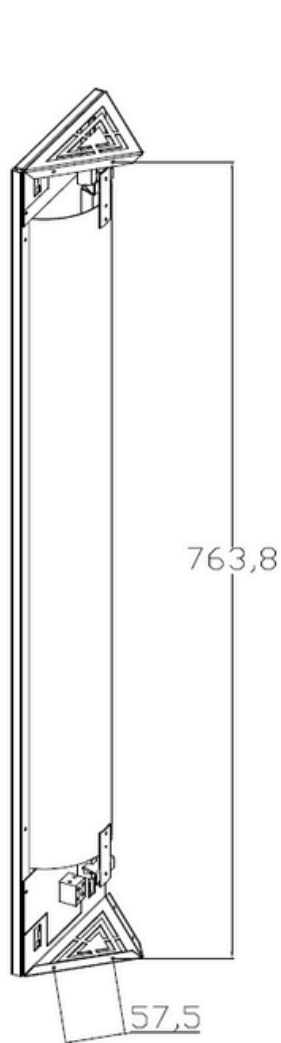
IRGLASS SPA Rozstaw otworów montaż narożny
